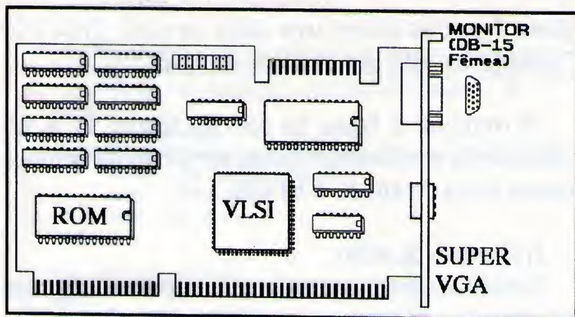
Figura 11 - placa SVGA de 16 bits.
